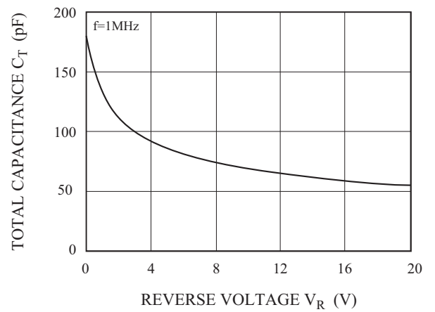
C_T - V_R
