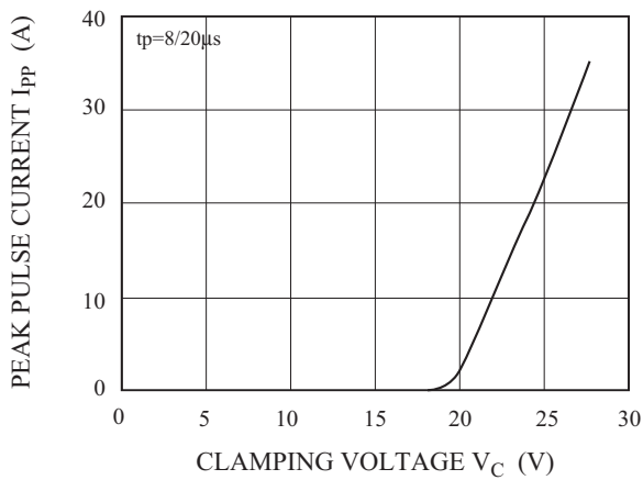
I_{pp} - V_C
