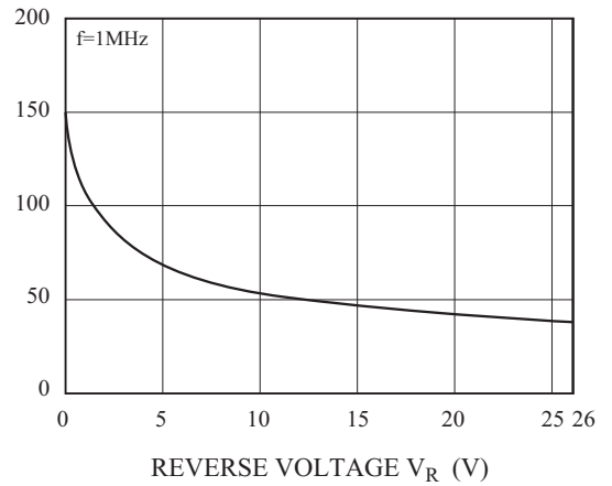
C_T - V_R
